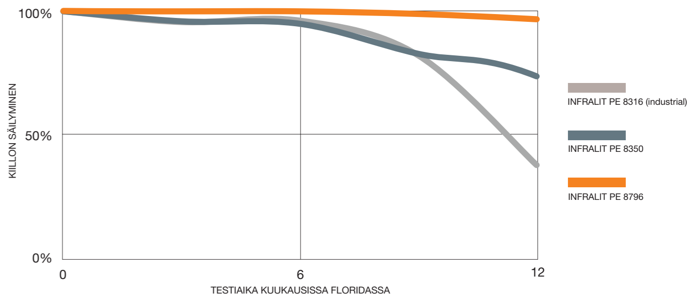
Tyypillinen kiillon säilyminen Florida -testissä (Testilevyjen suunta etelään, kallistus 5°)
